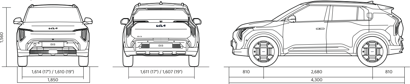
Afmetingen GT-Line
